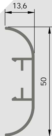
1007 Perfil de Remate
