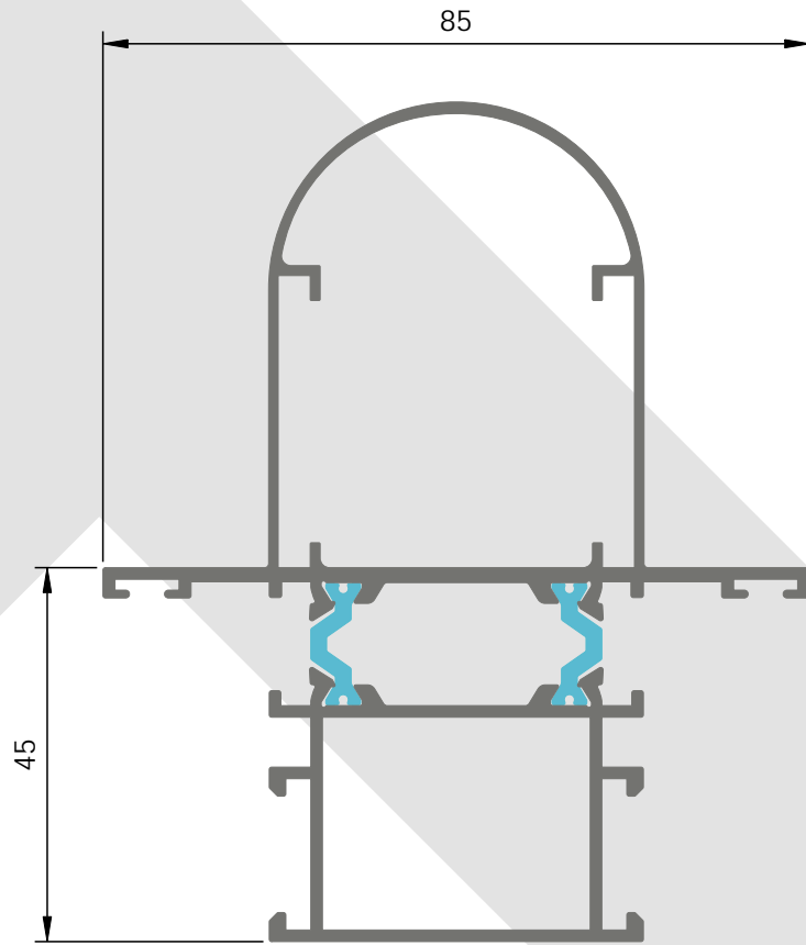
PT-16 Montante Reforçado
