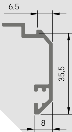
1001 Perfil de Remate
